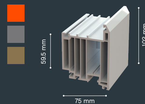
R003FD Flush Door Sash
