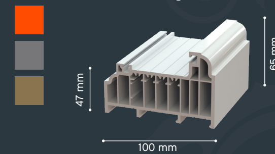
R010 Door Frame/Fixed Light Frame
